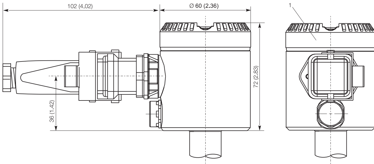
Рис. 2: Размеры указаны в мм (дюймах) - с опциями 1 Крышка корпуса при опциональном ЖК-дисплее
