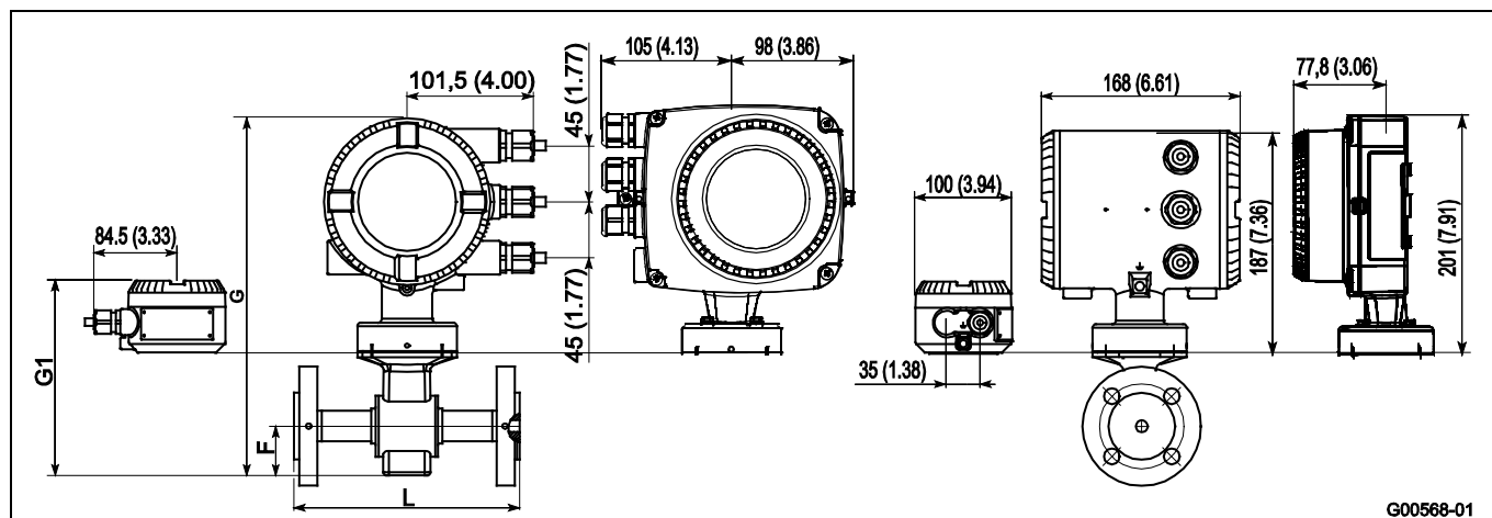
Рис. 33: размеры указаны в мм (дюймах)
