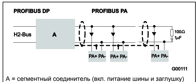
Рис. 15: пример подключения по интерфейсу PROFIBUS PA
