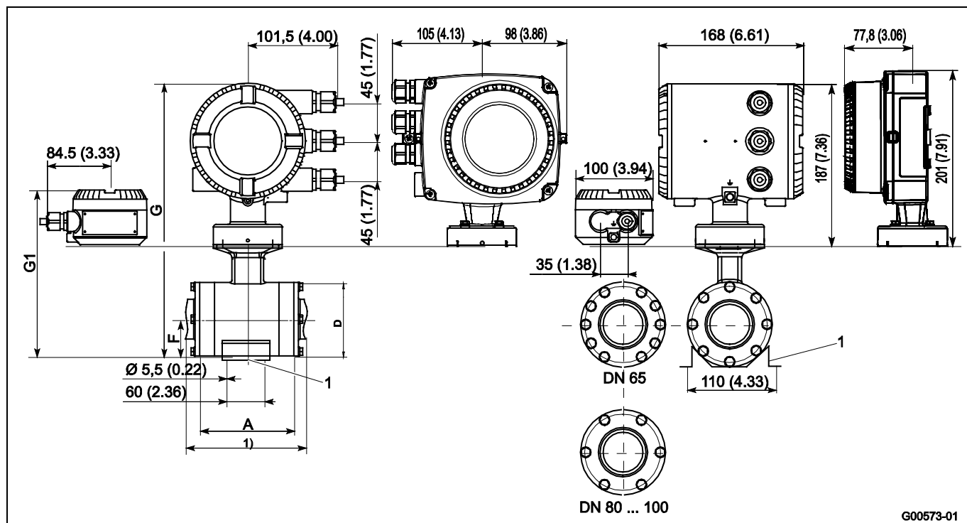
Рис. 38: Размеры в мм (inch)
