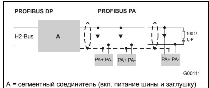
Рис. 19: пример подключения по интерфейсу PROFIBUS PA
