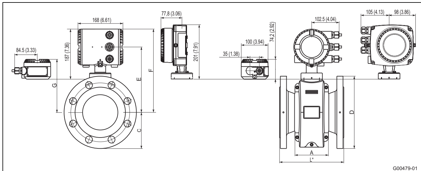
Рис. 39: размеры указаны в мм (дюймах)
