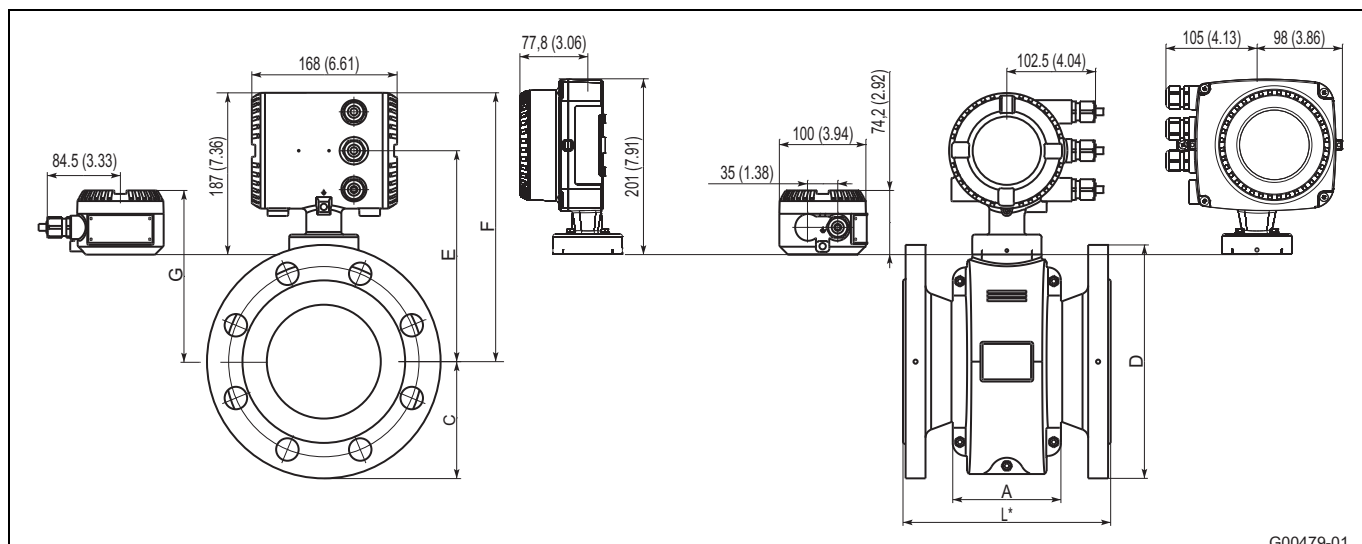
Рис. 42: размеры указаны в мм (дюймах)
