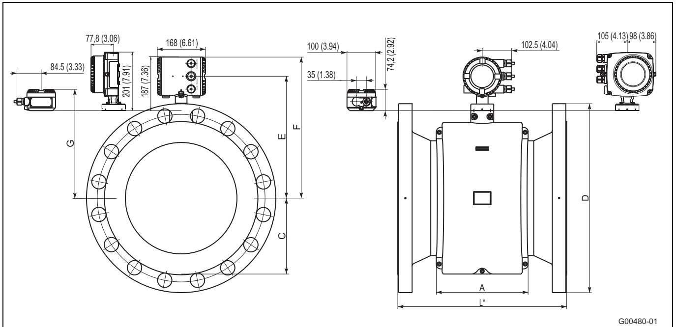
Рис. 40: размеры указаны в мм (дюймах)
