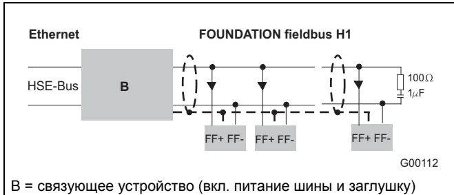
Рис. 20: пример подключения по интерфейсу FOUNDATION fieldbus
