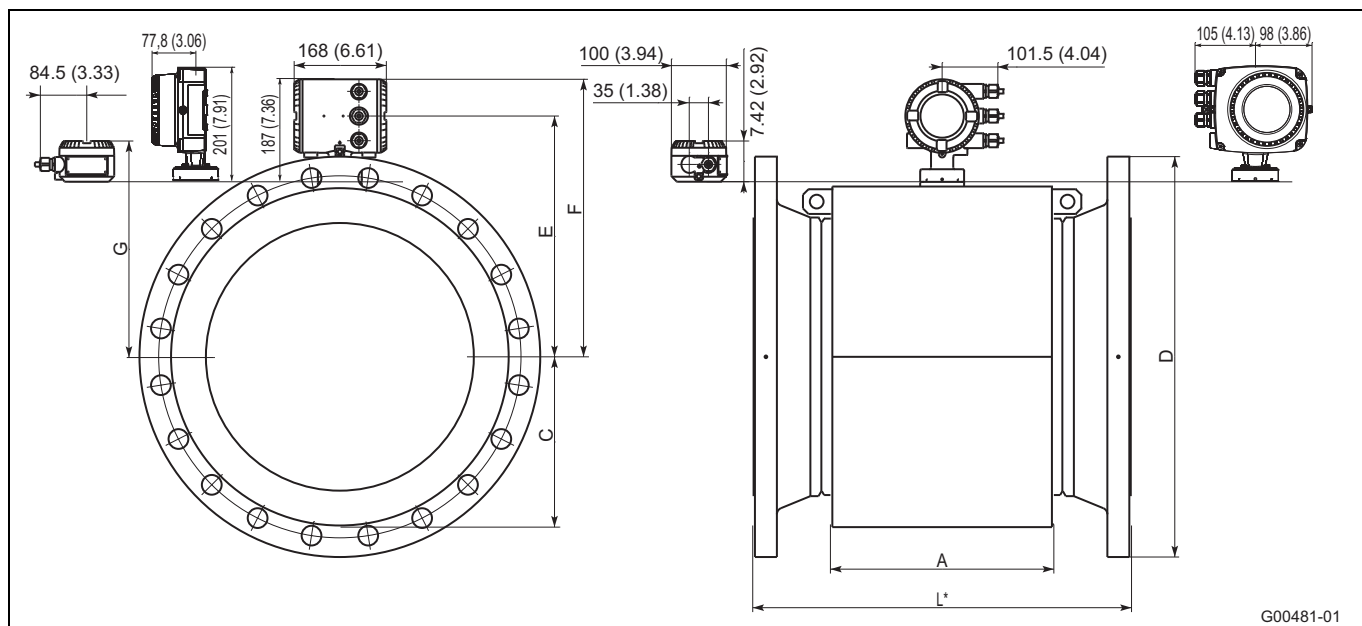
Рис. 41: размеры указаны в мм (дюймах)
