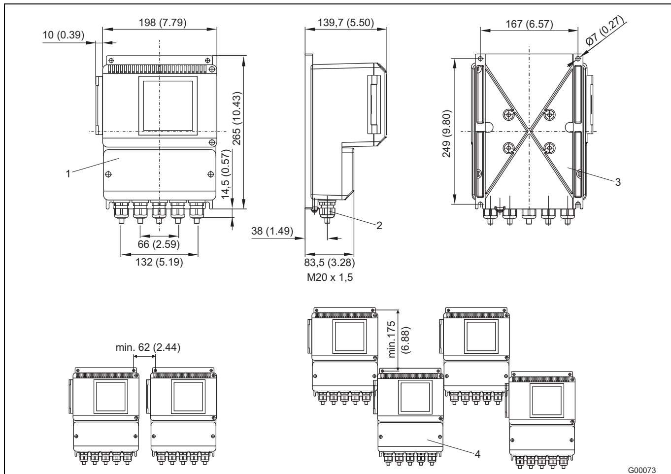
Рис. 44: размеры указаны в мм (дюймах)
