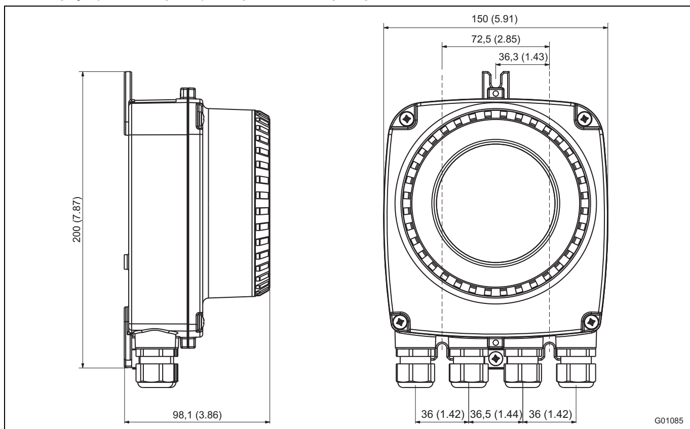
Рис. 46: размеры указаны в мм (дюймах)
