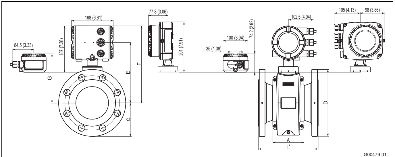
Рис. 43: размеры указаны в мм (дюймах)
