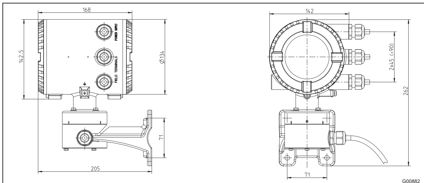
Рис. 45: размеры указаны в мм (дюймах)
