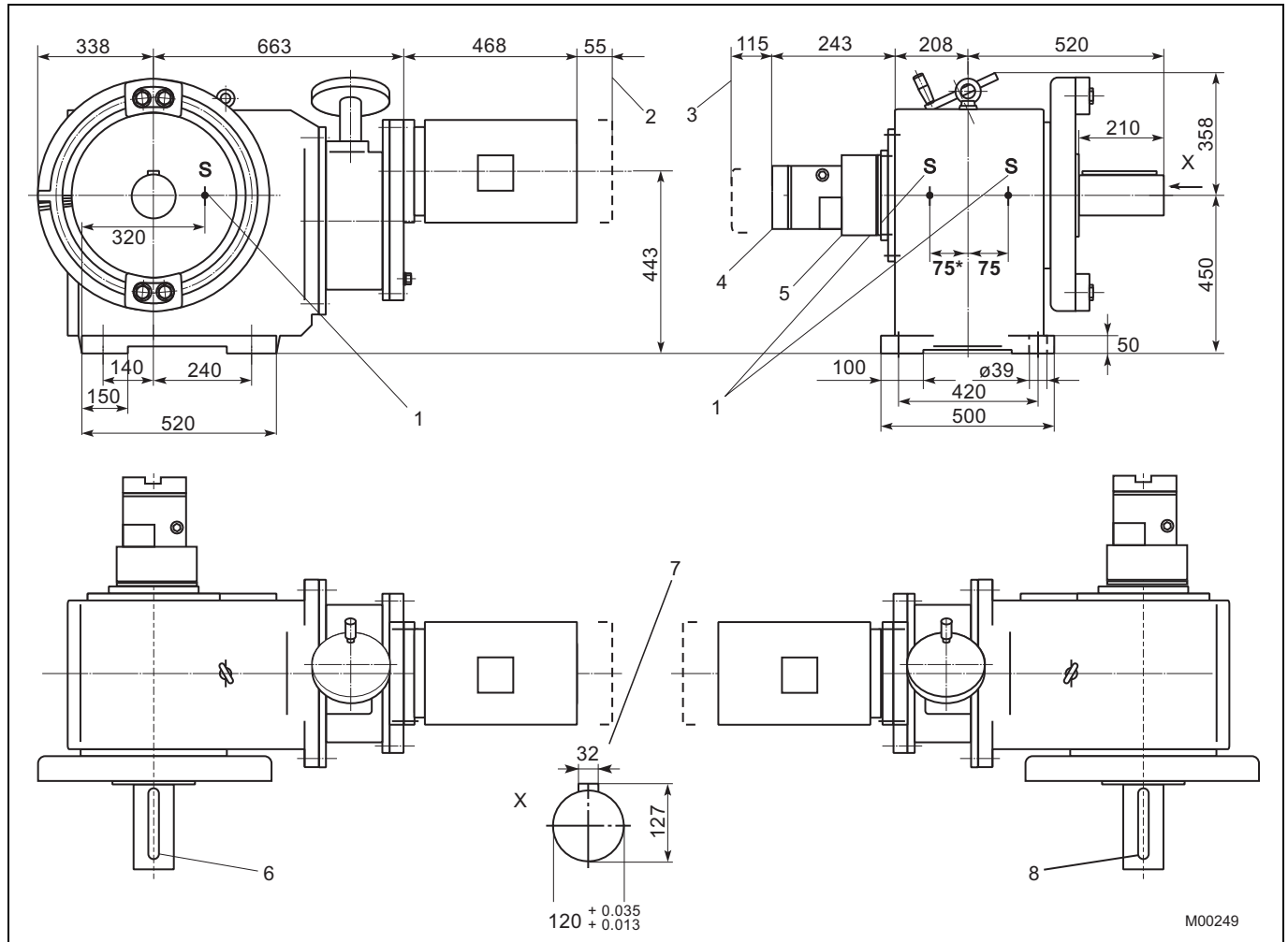
Рис. 5: габариты в мм
