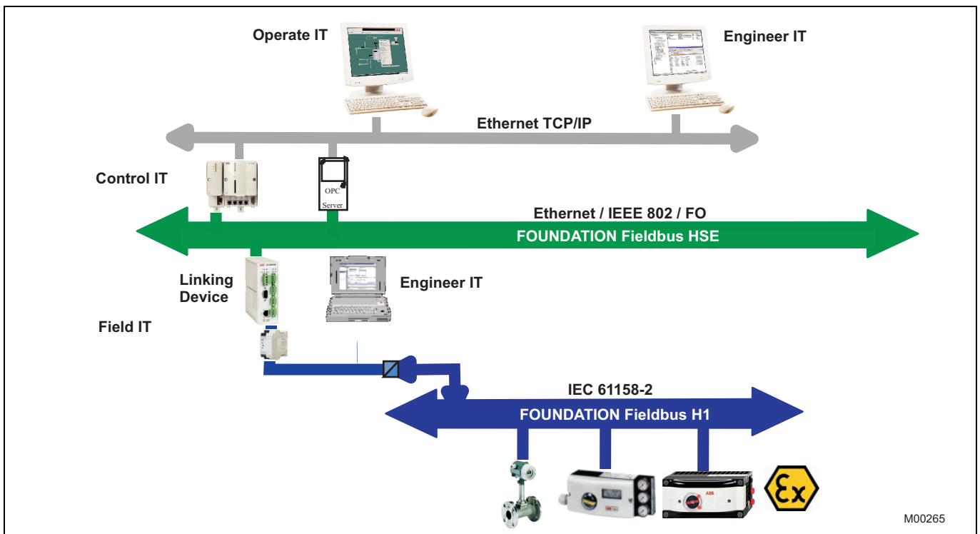
Рис. 5: Связь по шине FOUNDATION Fieldbus
