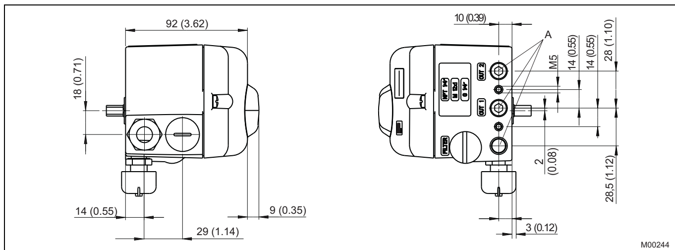
Рис. 10: Вид сбоку (слева направо)
