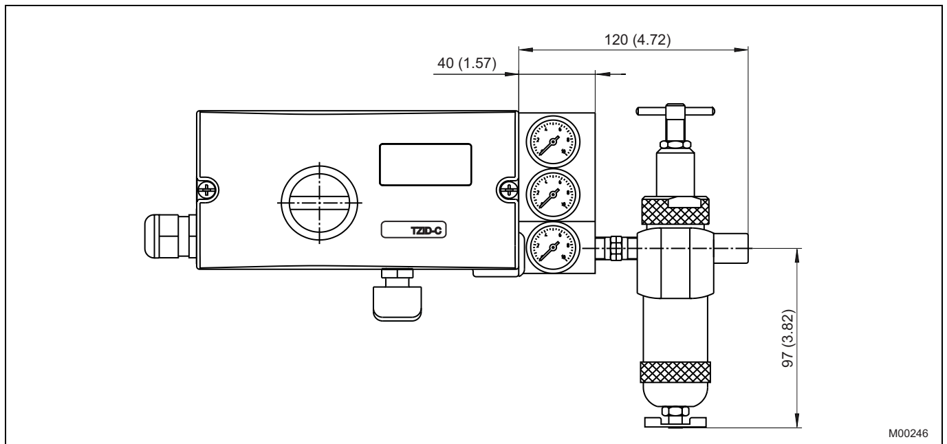
Рис. 12: Позиционный регулятор TZIDC-120 с установленным блоком манометров и фильтром-регулятором
