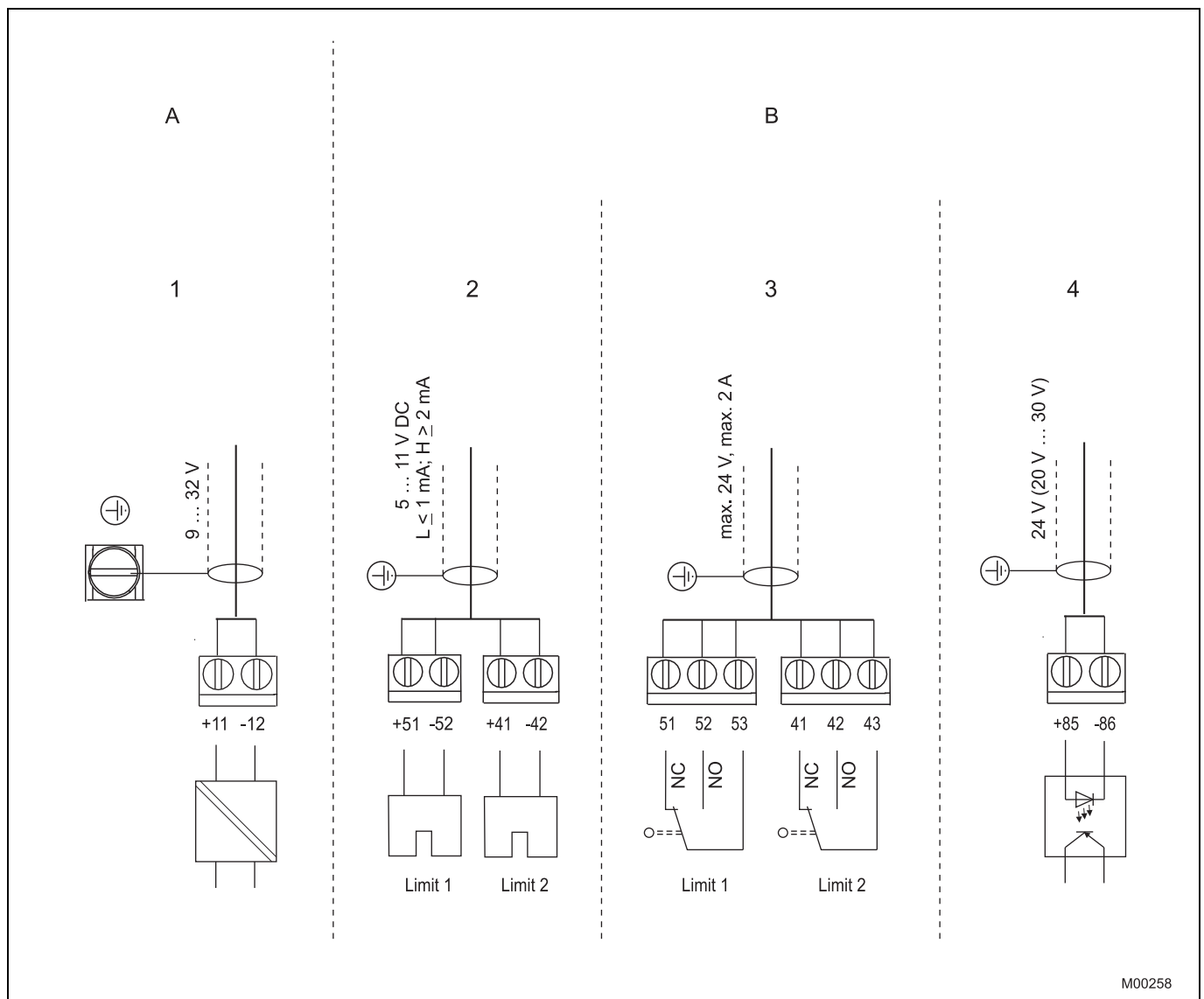
рис. 7: Расположение выводов
