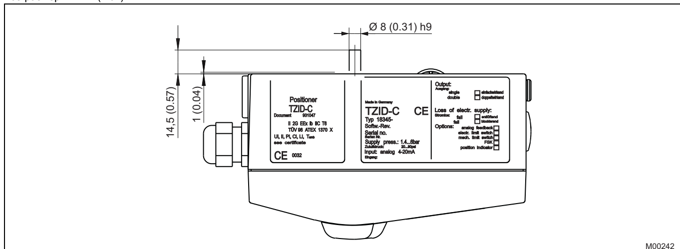
Рис. 8: Вид сверху
