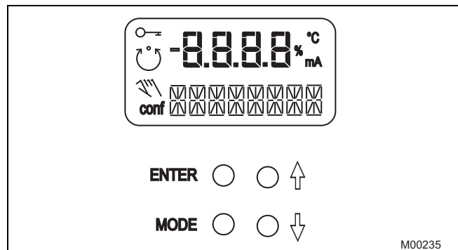
Рис. 4: Органы управления и индикации регулятора TZIDC-120
