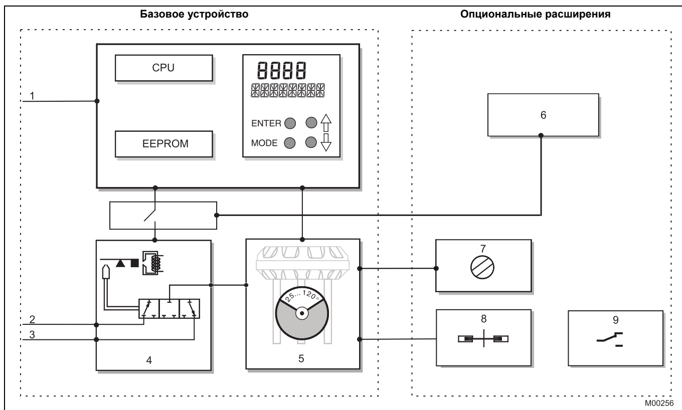
рис. 1: Схематическое изображение TZIDC-120
